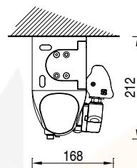
Montaje a techo
