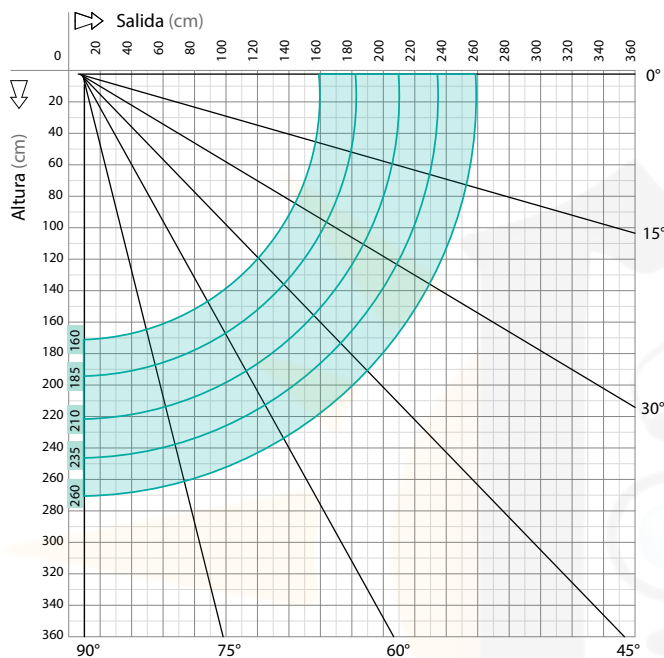
Diagrama de proyección - Montaje a pared/techo
