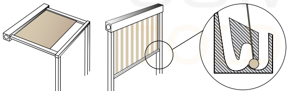
SISTEMA DE ENGANCHE/DESENGANCHE
