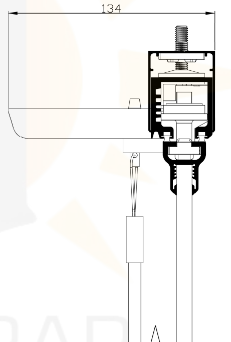
Sección vertical, con compensador superior e inferior
