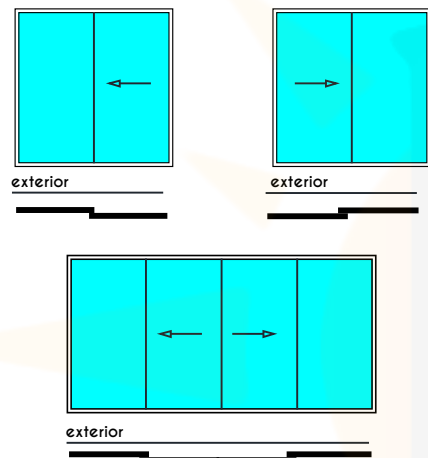
Configuraciones 2 Raíles
