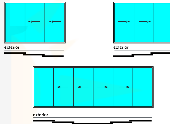
Configuraciones 3 Raíles
