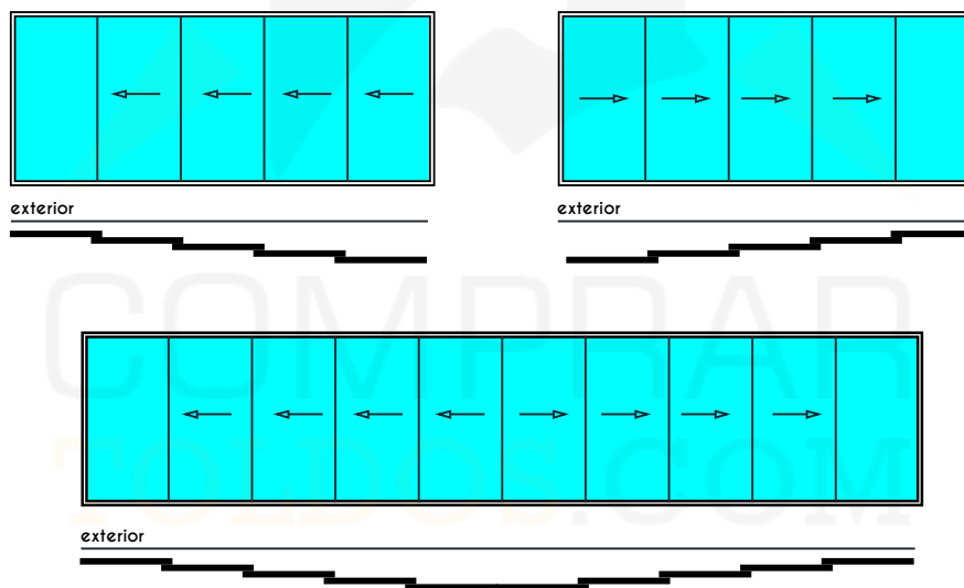
Configuraciones 5 Raíles
