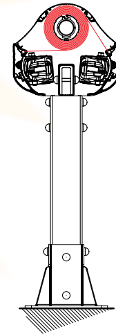
Sezione Section
