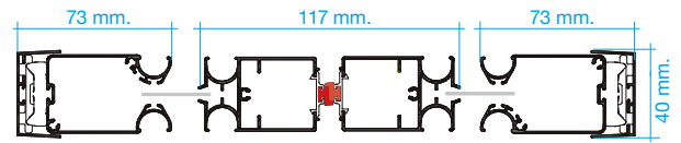
PUERTA DOBLE
