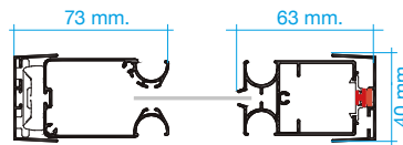
PUERTA ÚNICA
