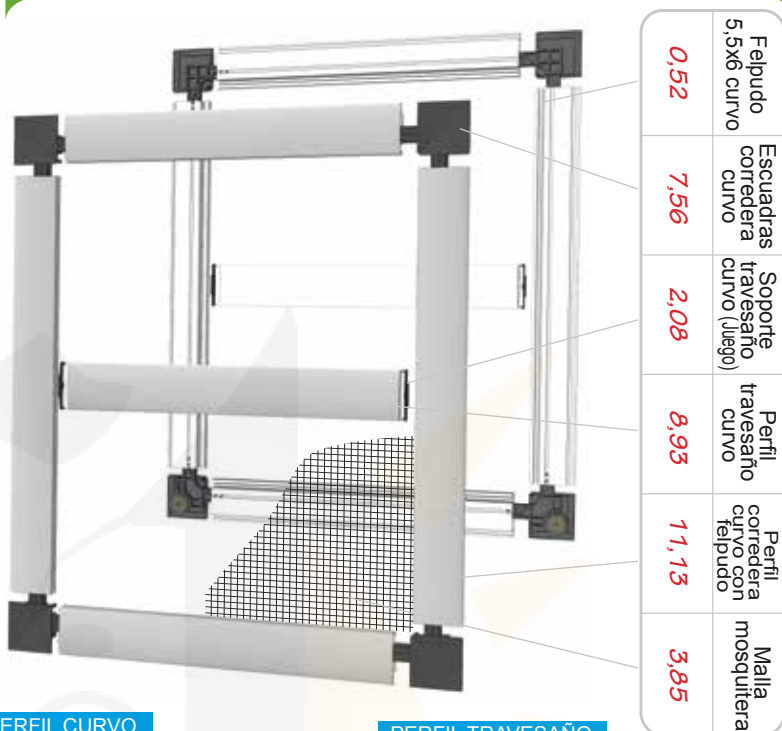
PERFIL TRAVESAÑO
