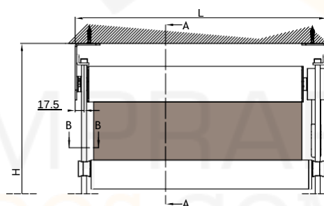
supporto a parete - wall bracket
