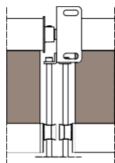
modulo doppio double module A-A
