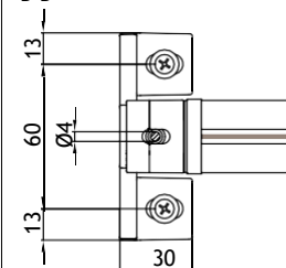
piedino a pavimento - floor bracket B-B
