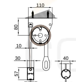
GA Posteriore - GA back A-A
