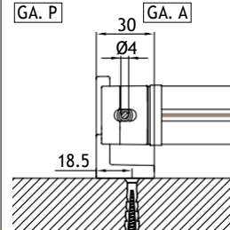
piedino a pavimento - floor bracket B-B
