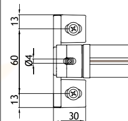
piedino a pavimento - floor bracket B-B
