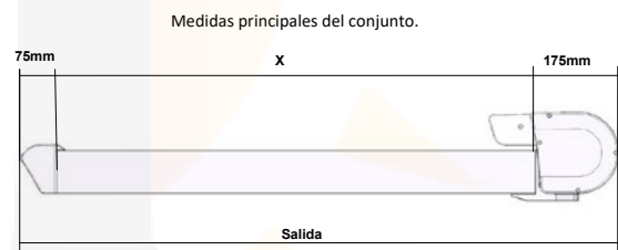
Medidas con KIT PIE VERANDA PRO
